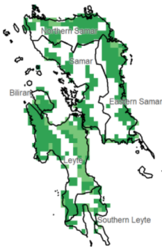
NDVI
