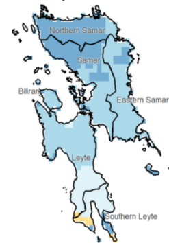
SPEI3 (Nov-Dec-Jan)
